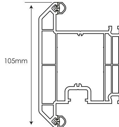
105mm Door T Sash 504635 / 584635
