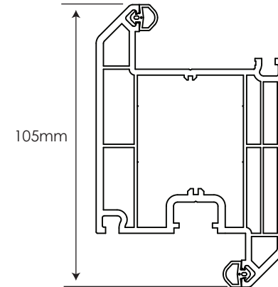
105mm Door Z Sash 504645 / 584645
