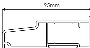
95mm Cill 504660 / 584660
