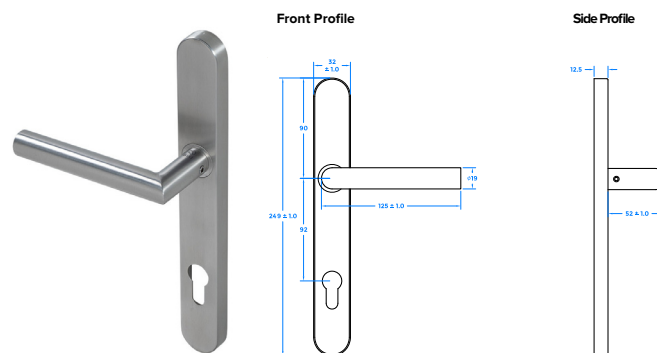
Mitre Lever Door Handle (Dual Sprung) - KM078
